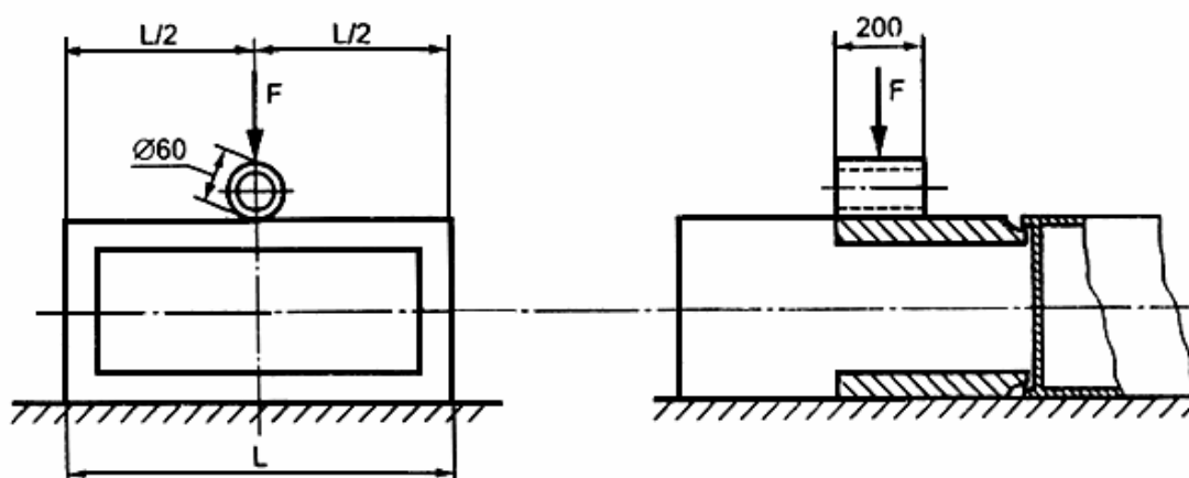
Рисунок 8 - Ударный элемент для проведения испытания по проверке устойчивости к механическим ударам, наносимым предметами с острыми кромками
