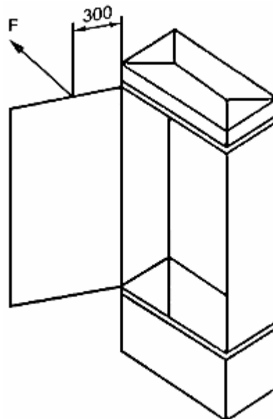
Рисунок 6 - Схема испытания по проверке сопротивления удару
