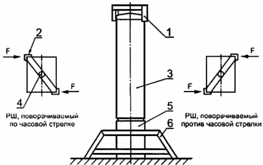
Рисунок 4 - Схема испытания по проверке устойчивости к ударной нагрузке
