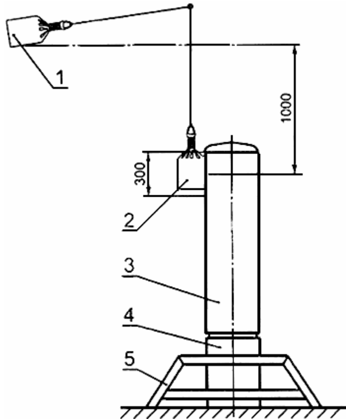
Рисунок 4 - Схема испытания по проверке устойчивости к ударной нагрузке
